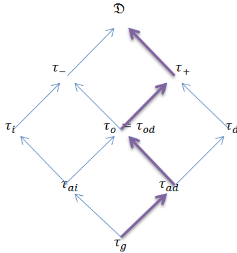
Diagrama 2: Una cadena de contenencias de topologías en los números reales.
