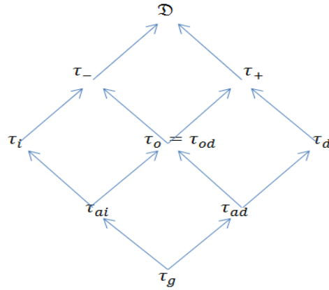
Diagrama 4: Topologías asociadas al orden en el conjunto del plano con el orden lexicográfico.
