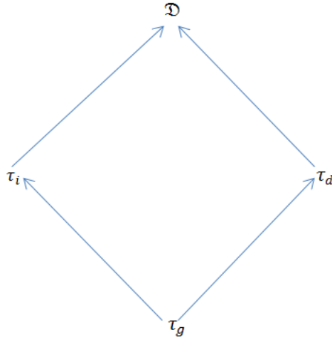
Diagrama 9: Topologías asociadas al orden en el conjunto del plano con el orden del producto.
